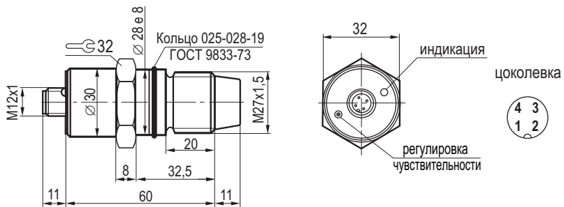
Габаритный чертеж
